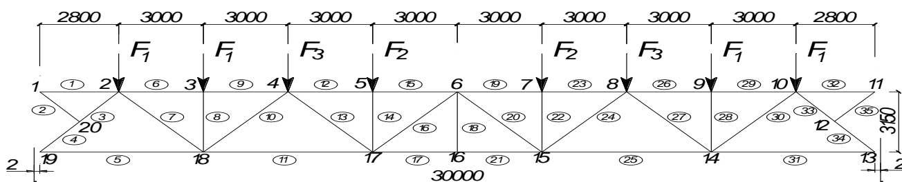
Рисунок 1 – К определению усилий в стержнях фермы
