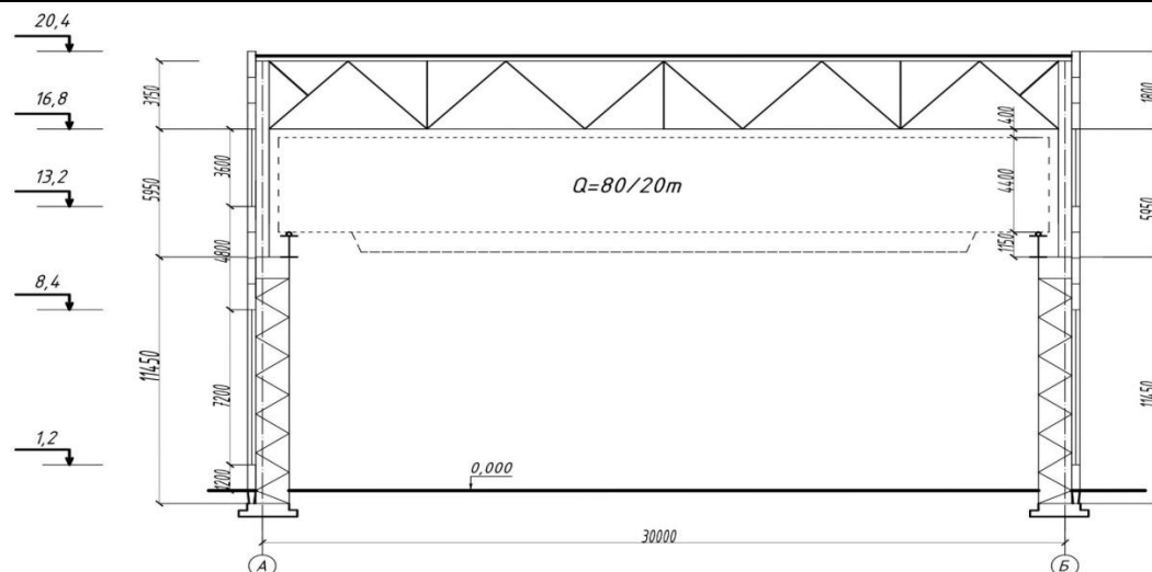
Рисунок 3 – Схема поперечной рамы
