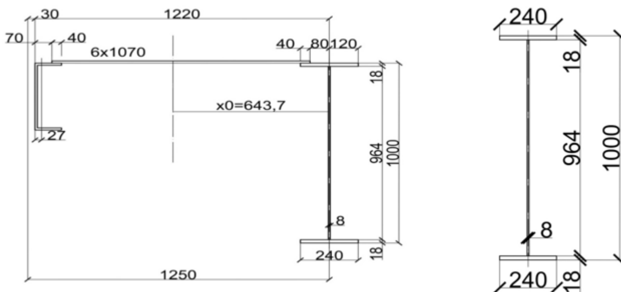
Рисунок 2 – Сечение подкрановой балки
