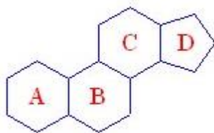
Стеран
