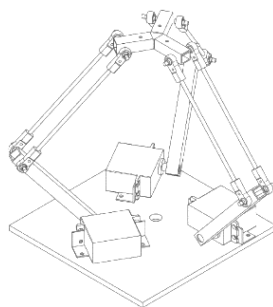
Рисунок 2 – Пример параллельного манипулятора
