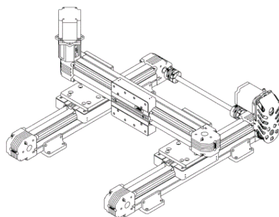
Рисунок 3 – Пример портального манипулятора
