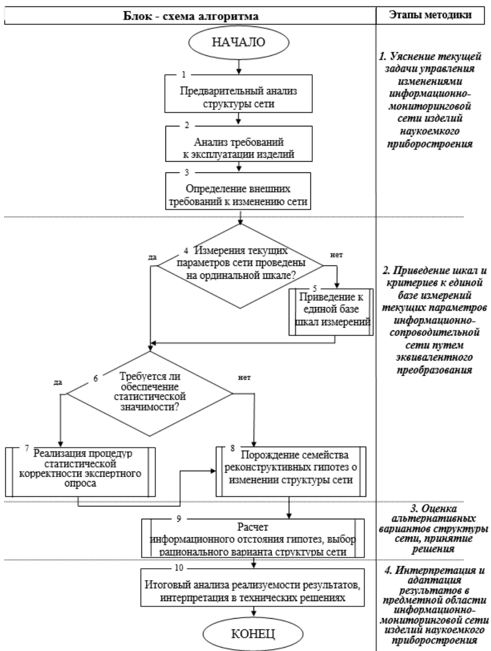
Рисунок – Обобщенный алгоритм реализации методики управления изменениями информационно-мониторинговой сети для продукции наукоемкого приборостроения Источник: разработано автором.
