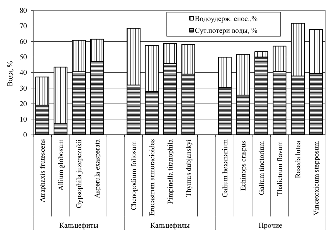
Рисунок 1 – Показатели водного режима травянистых растений различных групп
