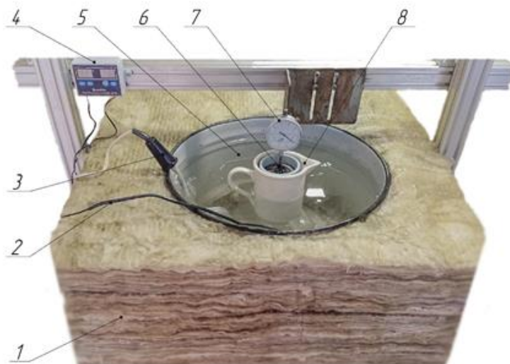
Рисунок 1 – Экспериментальная установка: 1 – Теплоизоляционный материал; 2 – Датчик температуры; 3 – Нагревательный прибор; 4 – Электронный регулятор температуры; 5 – Емкость с водой; 6 – Груз; 7 – Датчик ИЧ10; 8 – Емкость с серной кислотой.
