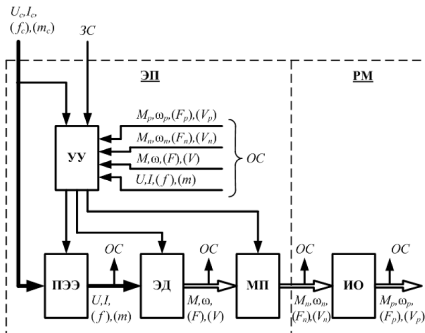
Рисунок 1 – Структурная схема электропривода механизма при работе ЭД в двигательном режиме.
